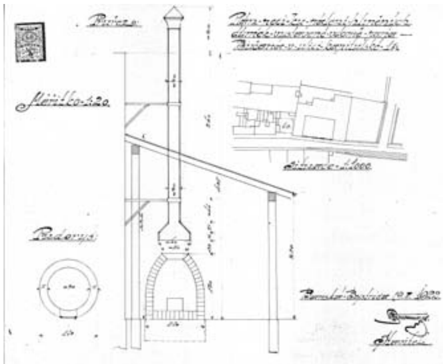
Plán pece na vypaľovanie hlinených fajok v Kapitulskej ulici č.19. Zdroj: Štátny archív v Banskej Bystrici MBB 173/1922, šk. č. 575.
