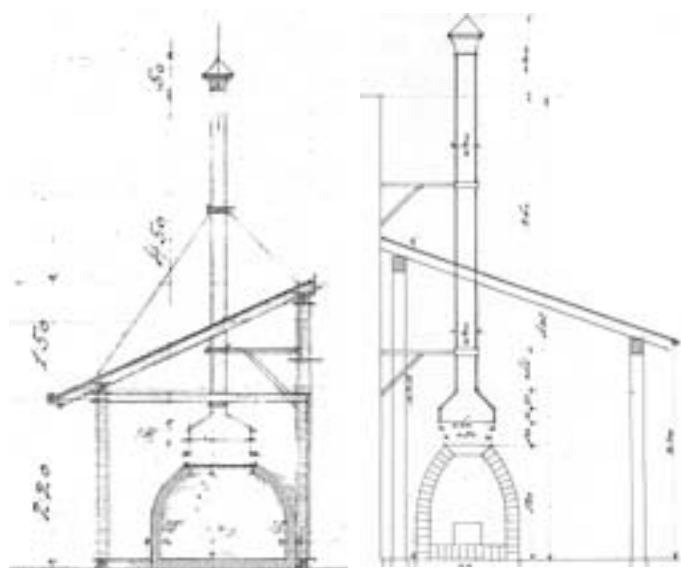
Porovnanie nákrasov pecí na vypaľovanie fajok: A – pec na Hor- nom predmestí, B – pec na Kapi- tulskej ulici.
